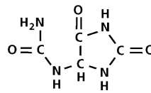
Allantoin
